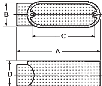
E Conduit Body
