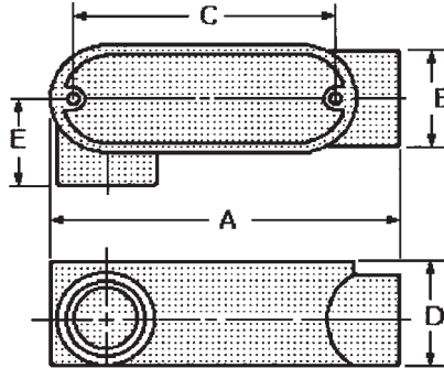
LR Conduit Body
