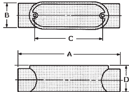
C Conduit Body
