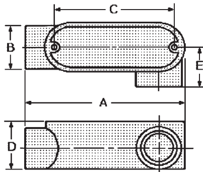
LR Conduit Body
