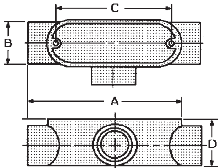
T Conduit Body
