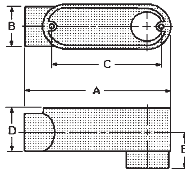
LB Conduit Body
